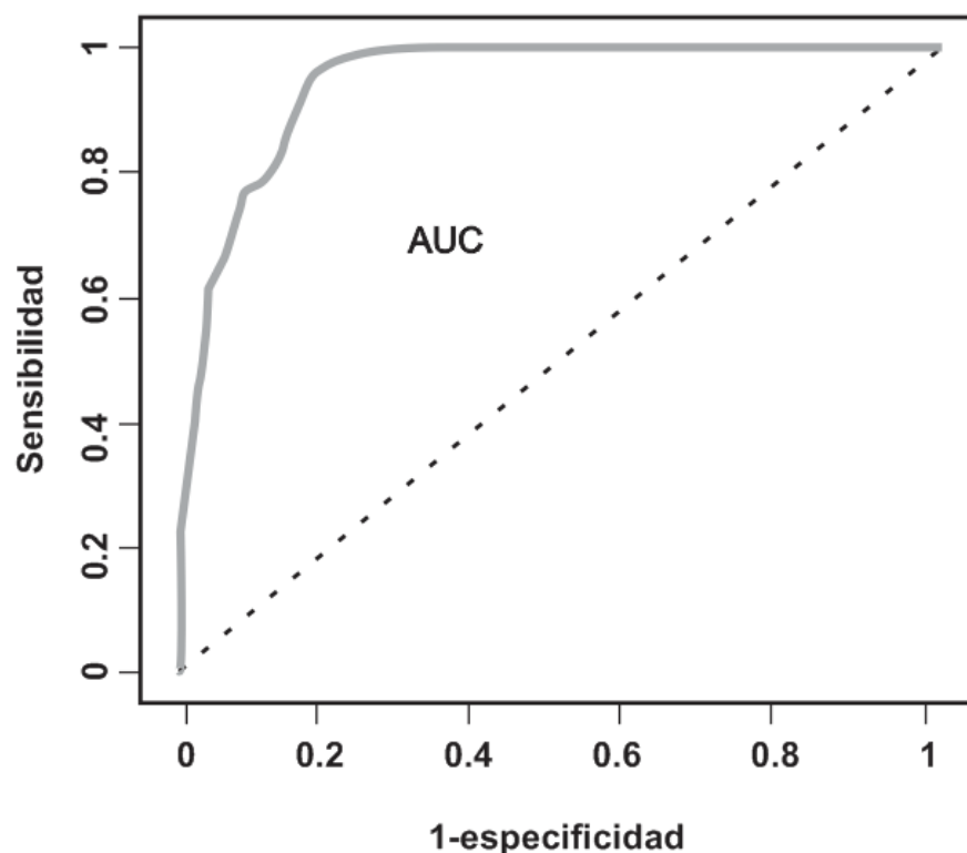
Fig. 2.6. Gráfica del AUC/ROC para medir el desempeño de un modelo. La línea gris representa los datos de instrucción con un AUC = 0.94. La línea negra intermitente representa una predicción basada en el azar AUC = 0.5.
