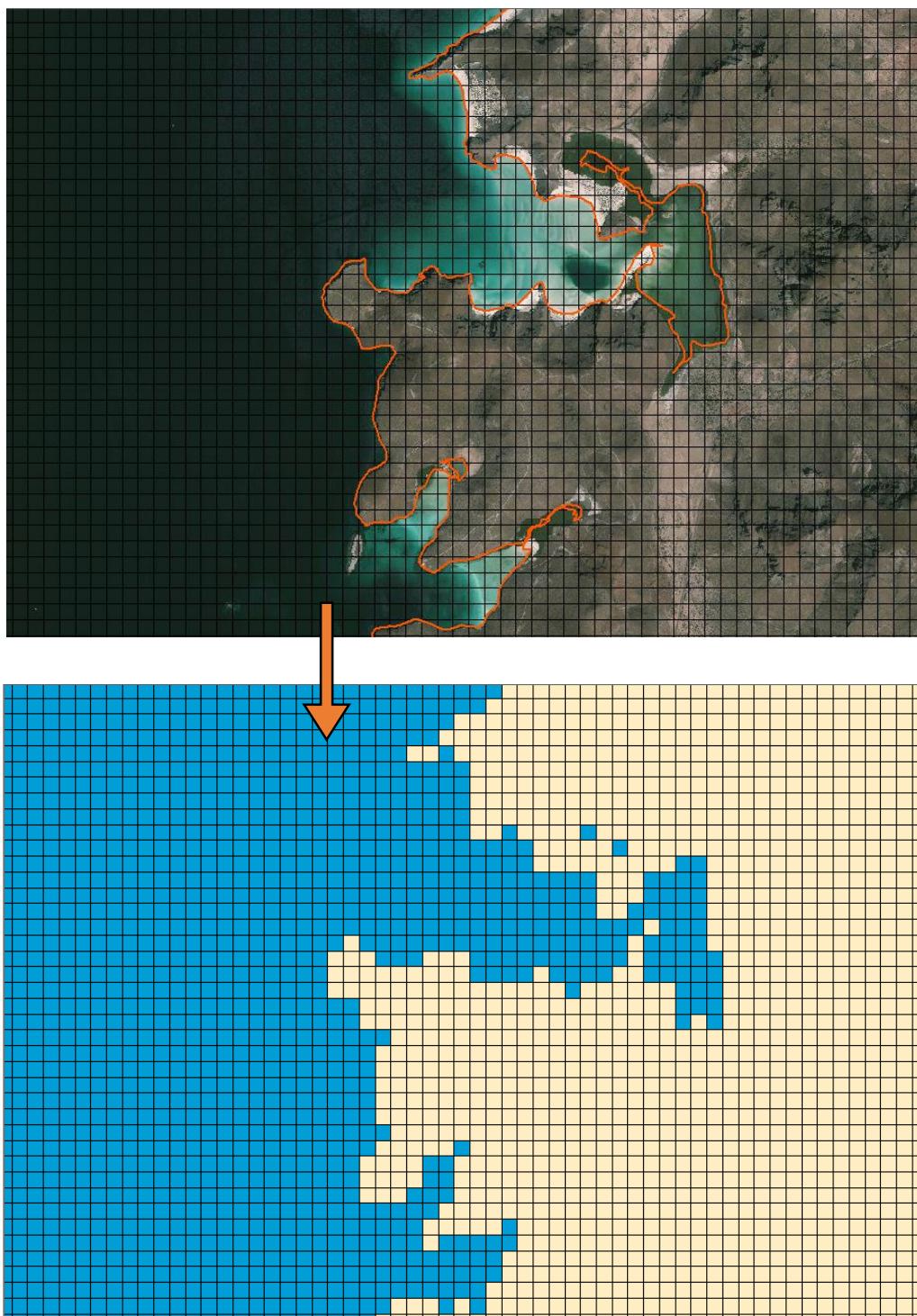
Fig. 4.2. Malla con cuadrantes de 100x100 m (1 ha) vista en una porción del mapa base. La línea anaranjada represena la línea de costa. Los pixeles en azul corresponden a la parte marina.
